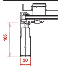
Montage im rechten Winkel zum Rollladen (A)
