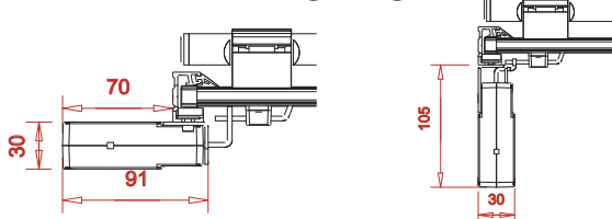
Montage parallel zum Rollladen (A)
