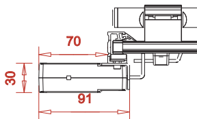
Montage parallel zum Rollladen (A)
