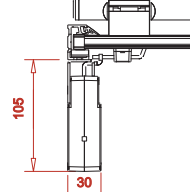
Montage im rechten Winkel zum Rollladen (A)
