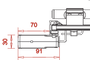
Montage parallel zum Rollladen (A)
