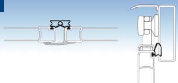
Dichtsystem / Sealing system
